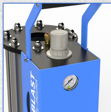
Réglage de pression de 0,5 à 8 bars avec manomètre pour une lecture simplifiée
