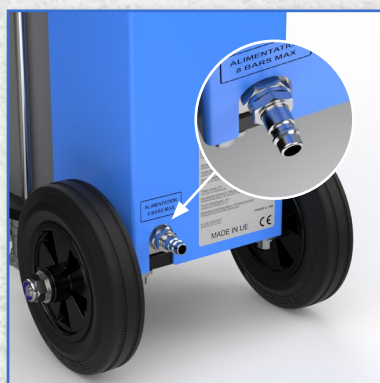
Alimentation en air comprimé via un raccord de type coupleur européen
