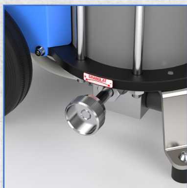
Vis de débit d'abrasif pour un réglage précis et rapide
